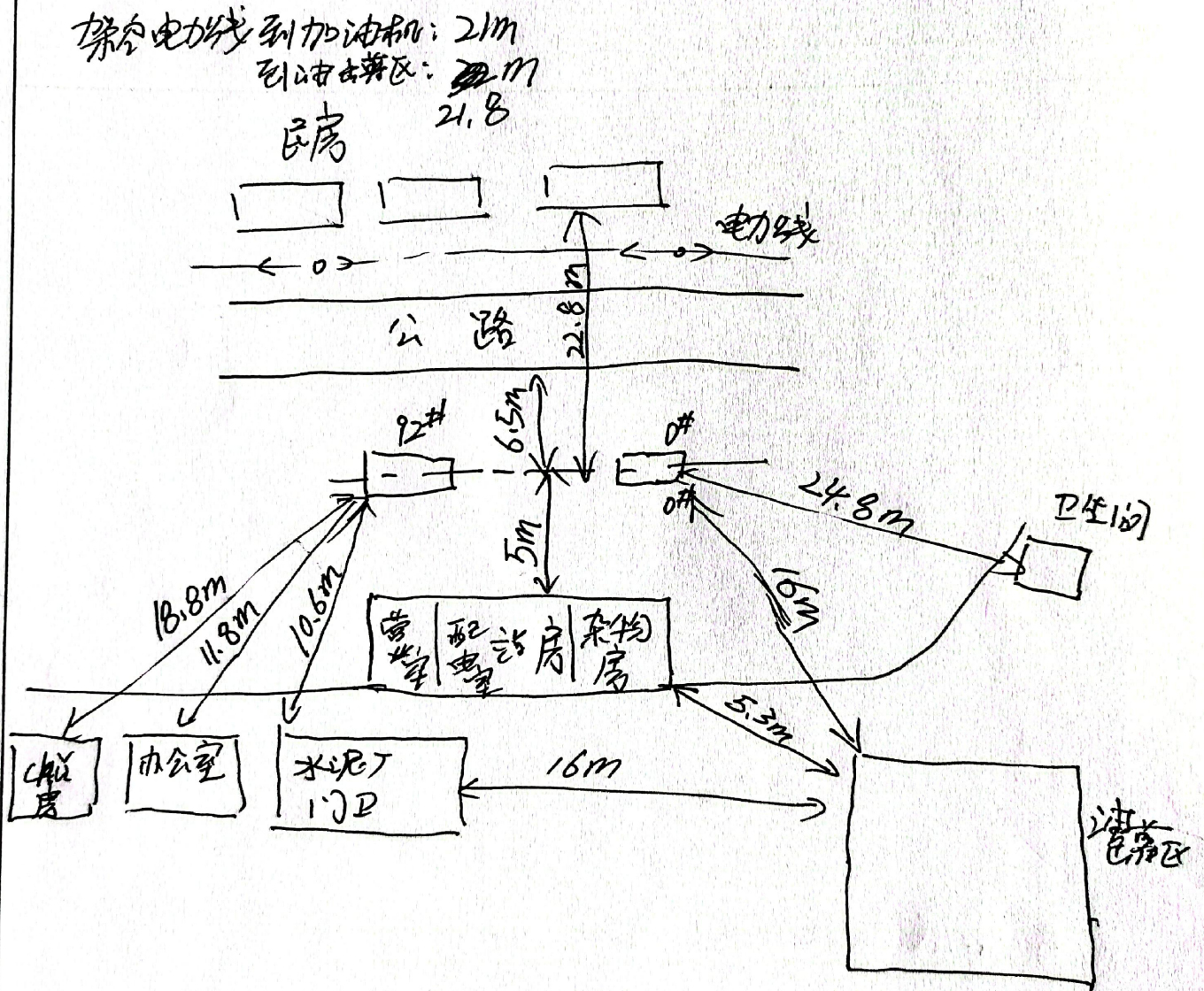
生产区域平面布置示意图
